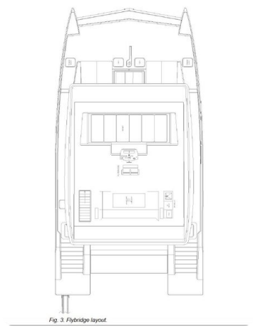
Fig. 3. Flybridge layout.
